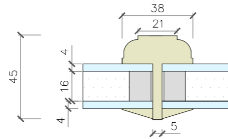
38/9 Ovolo Glazing Bar
