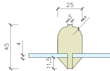
25/5 8.5mm radius Ovolo
