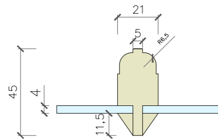
21/5 6.5mm radius Ovolo
